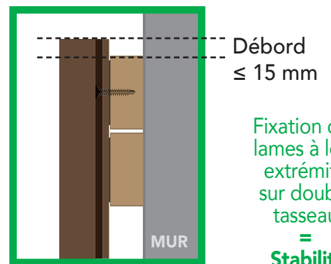
Vue du côté Pose verticale avec double tasseaux aux jonction des lames
