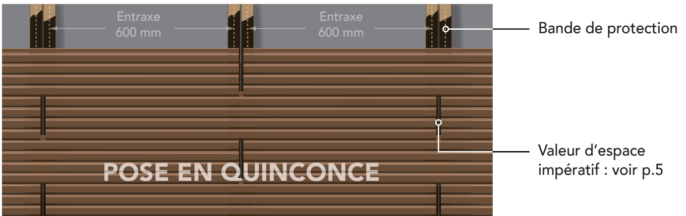
Fixation des lames à leur extrémité sur un tasseau = Stabilité
